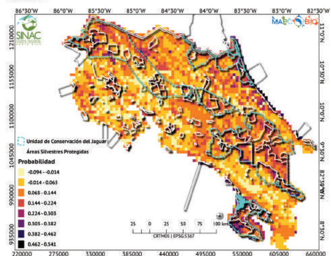
Modelo svm
