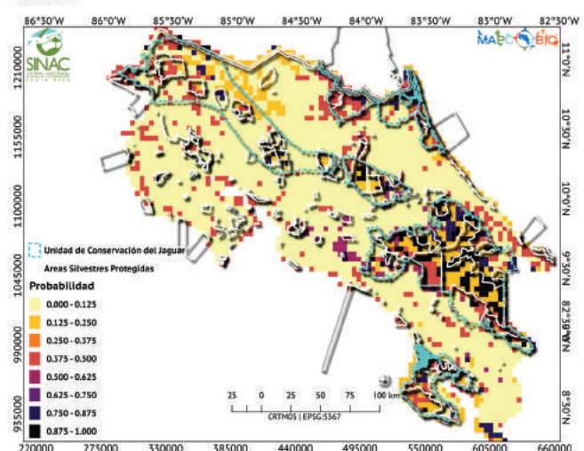
Modelo cart
